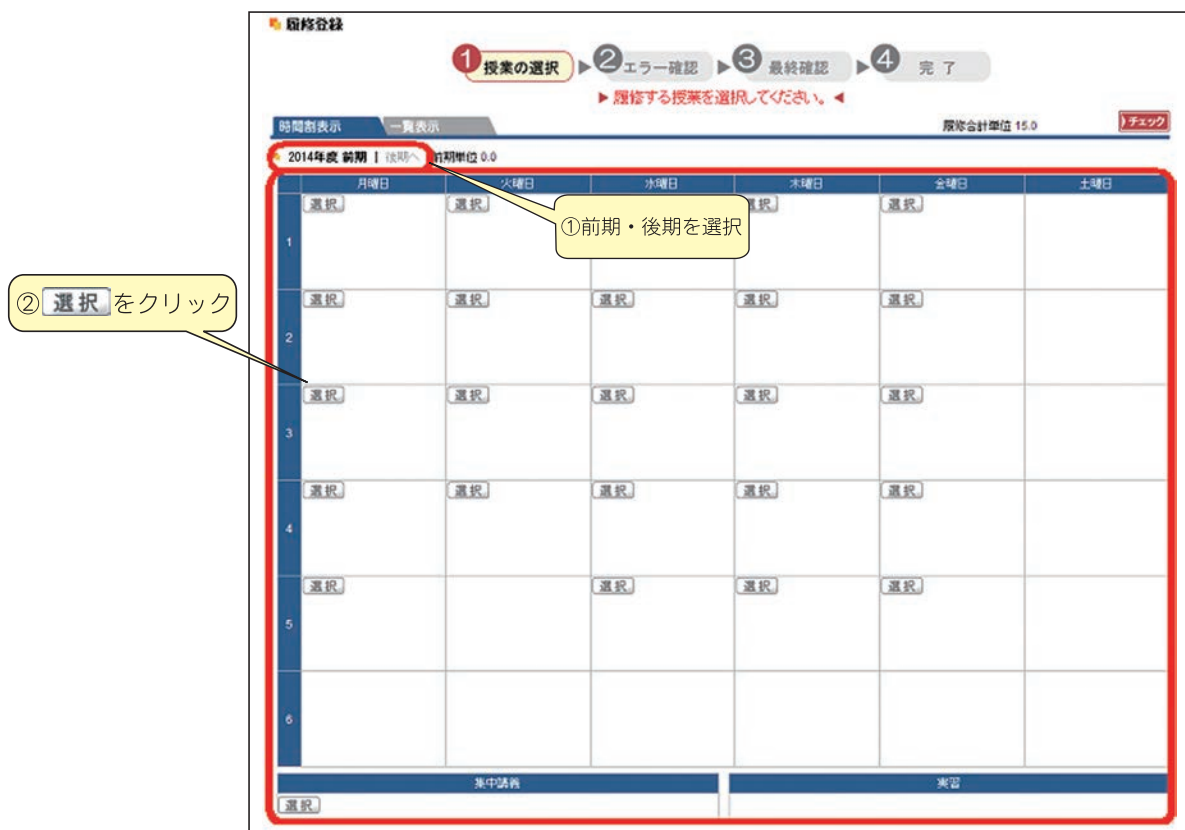
図2 履修登録画面
